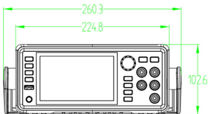
正视图
