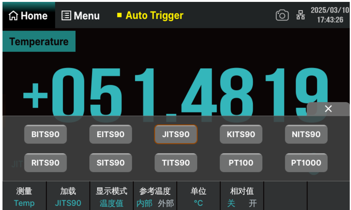
图 7-21 传感器类型选择界面
