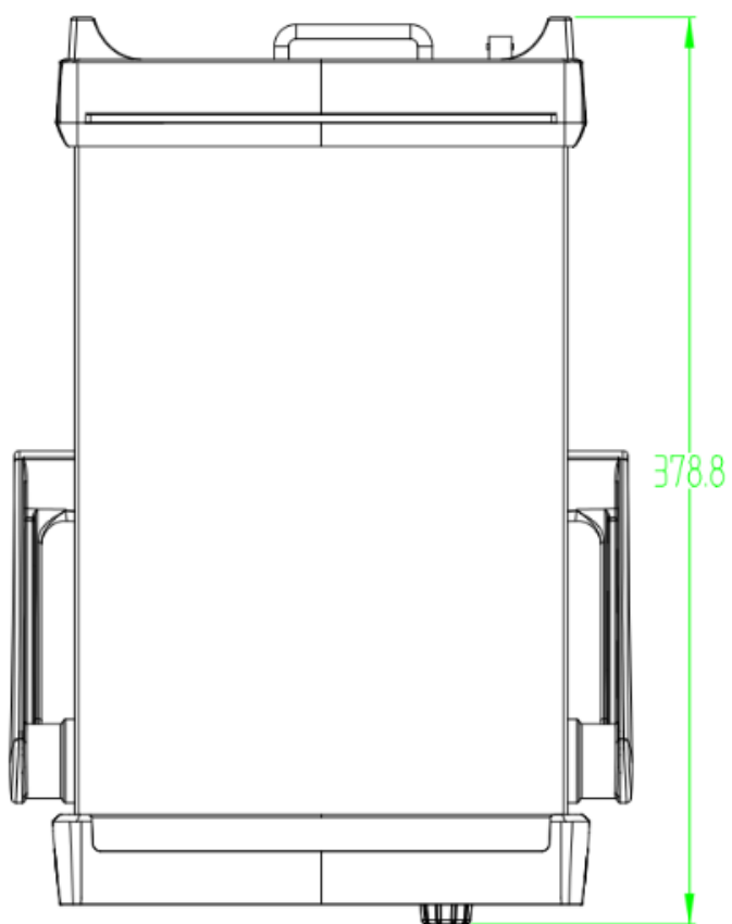
俯视图
