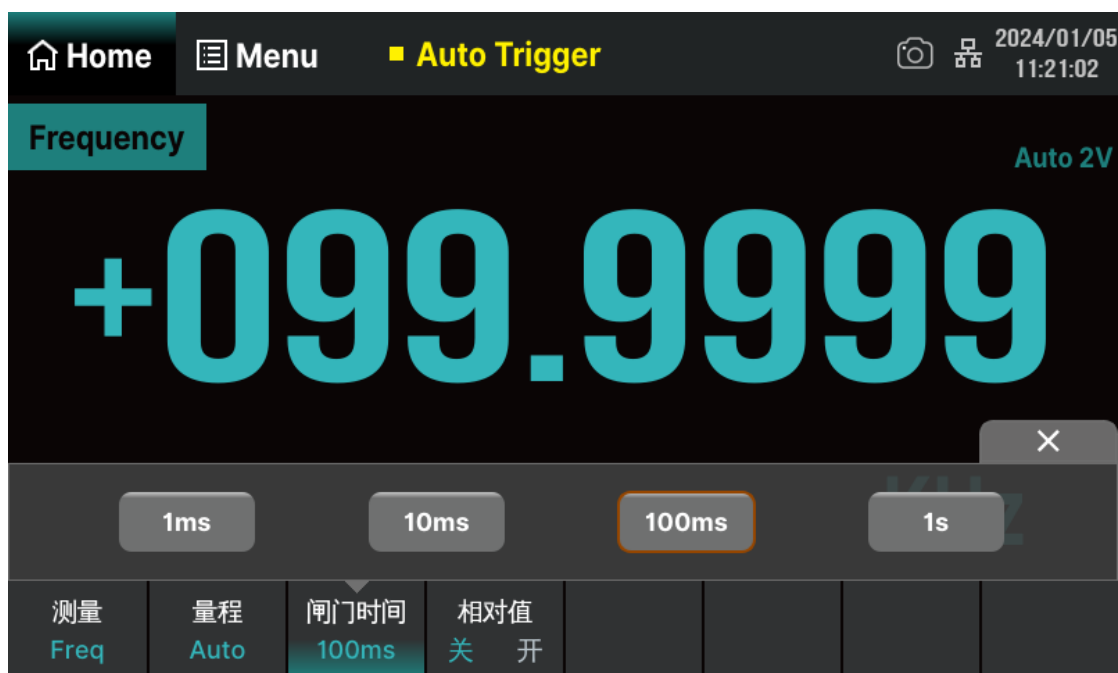
图 7-8 设置闸门时间
