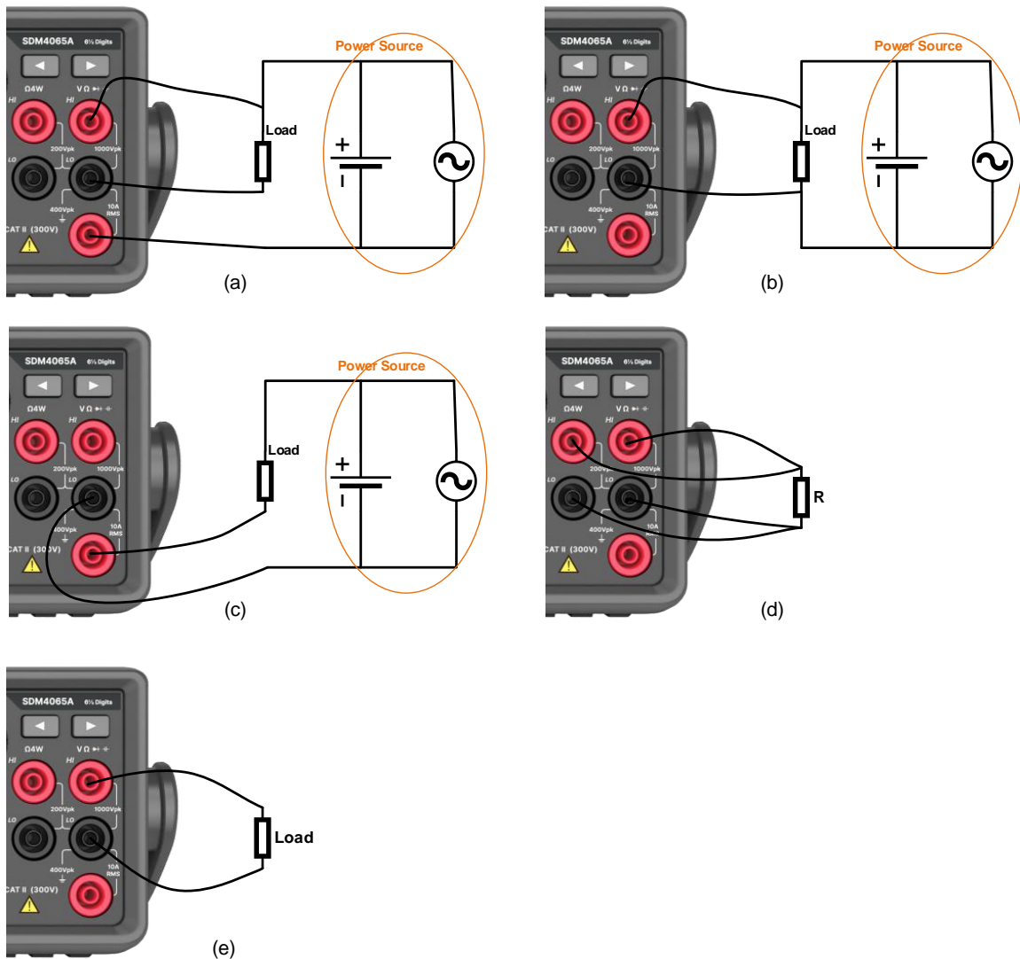
图 7-31 接线示例
