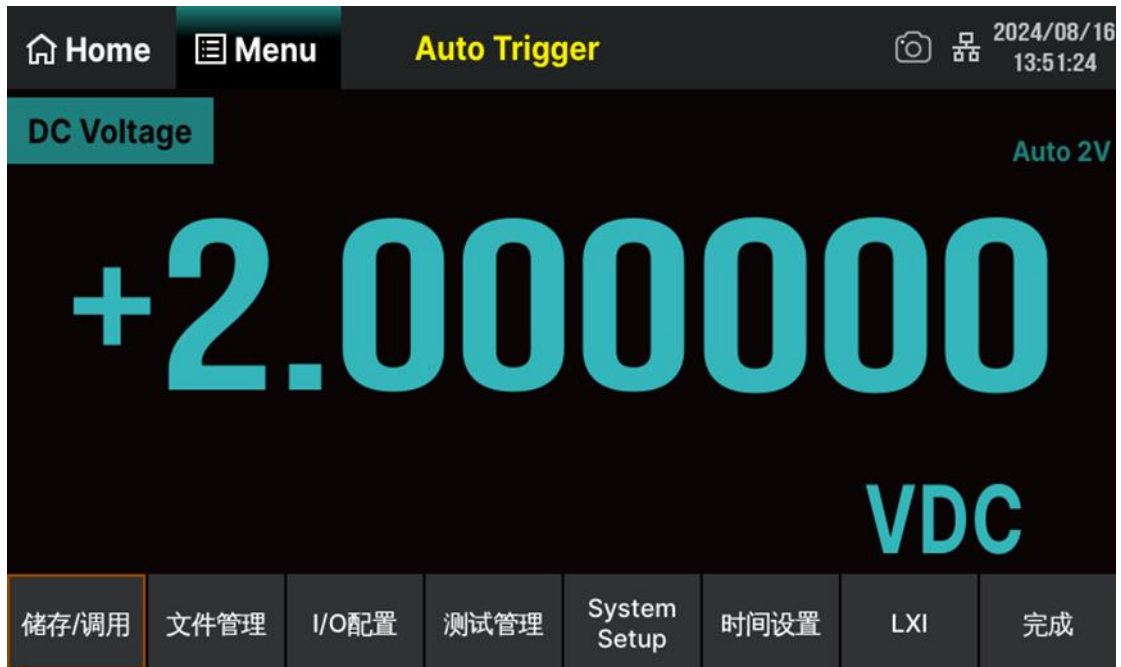
图 7-32 辅助功能设置界面
