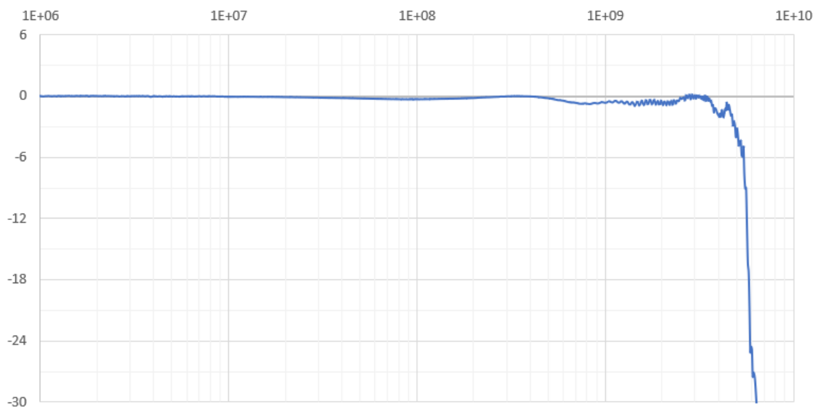
DRP-45 频响曲线
