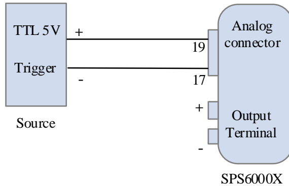
图 9-5 外部控制输出/关闭
