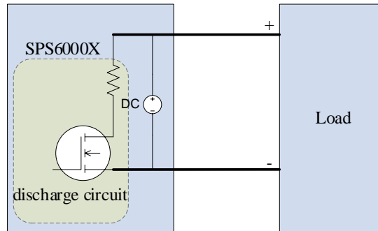
泄放电路
