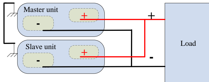
图 9-2 并联输出端口连接示意图
