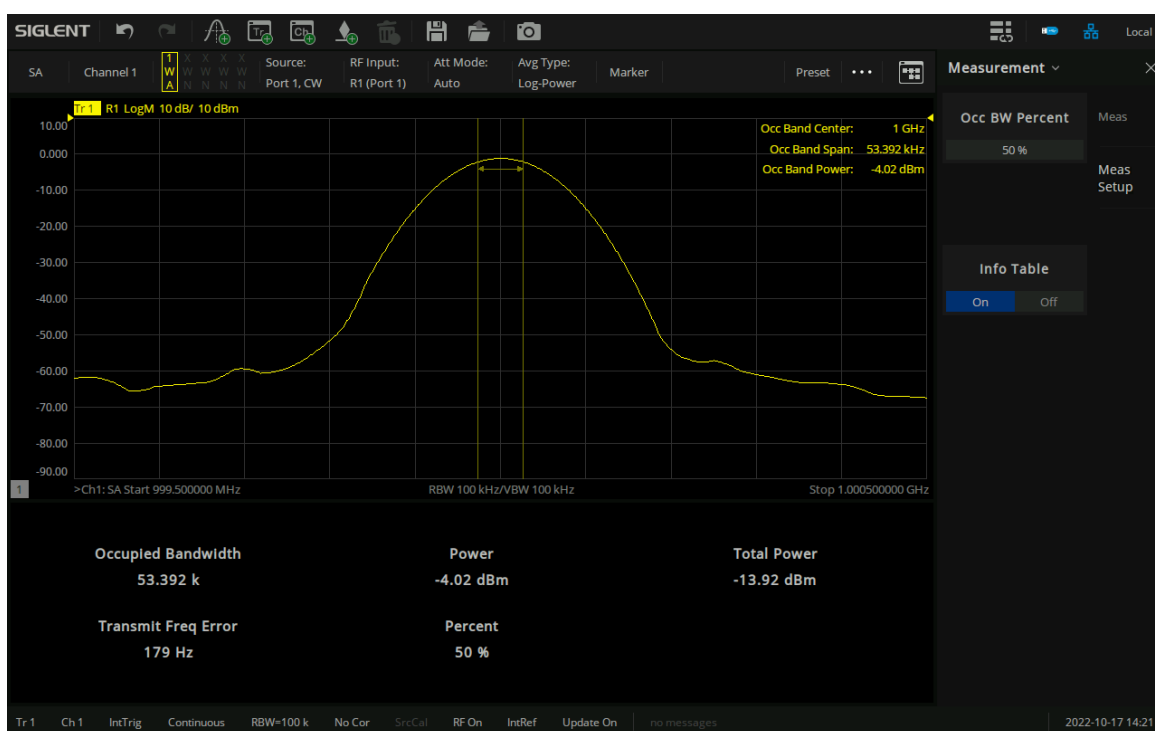
图 11-11-15 Occupied BW 测量界面
