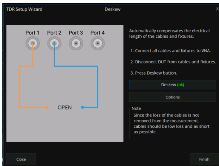
图 10-4 TDR 延时补偿校准向导
