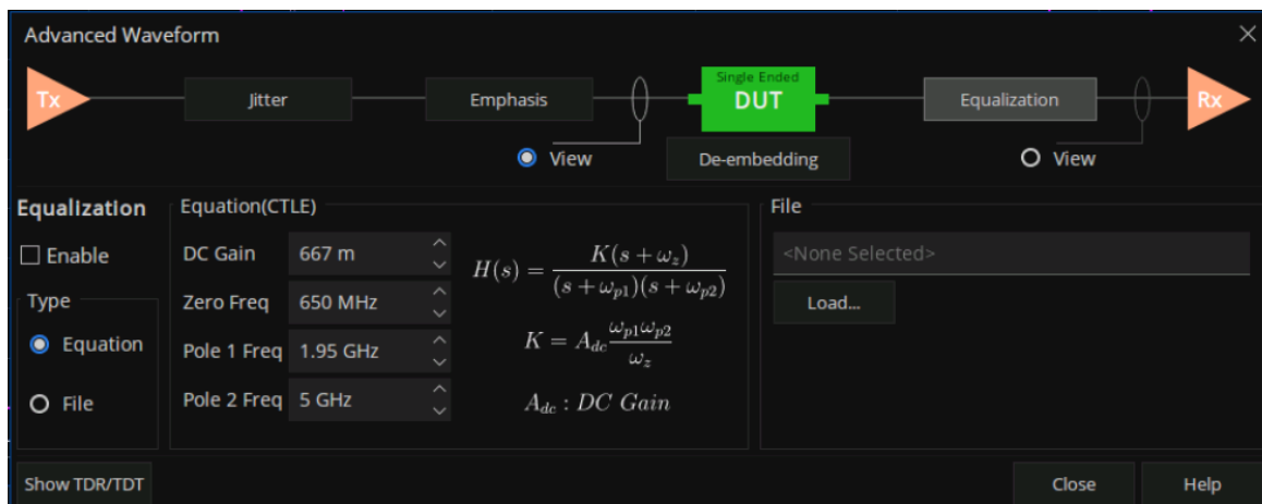
图 10-18 TDR 均衡设置
