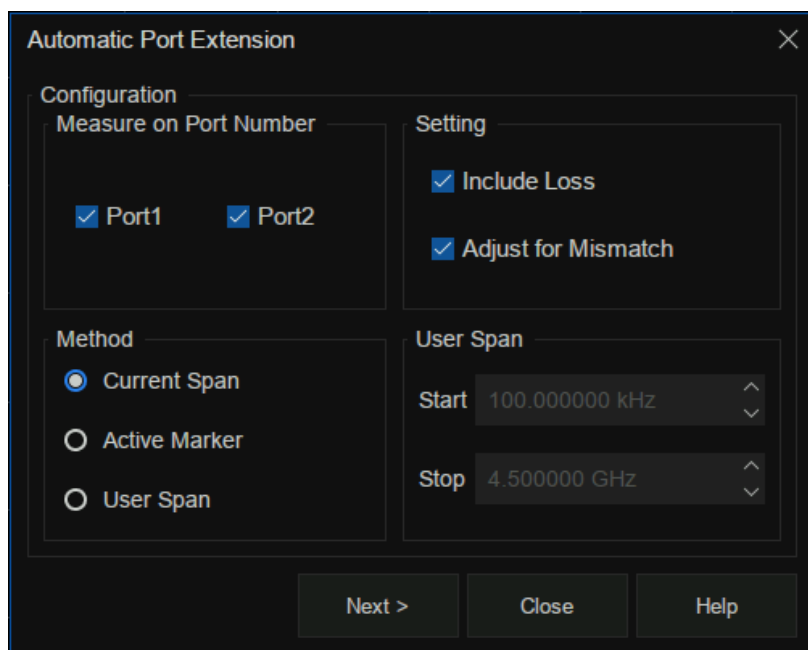
图 7-6 自动端口延伸设置界面
