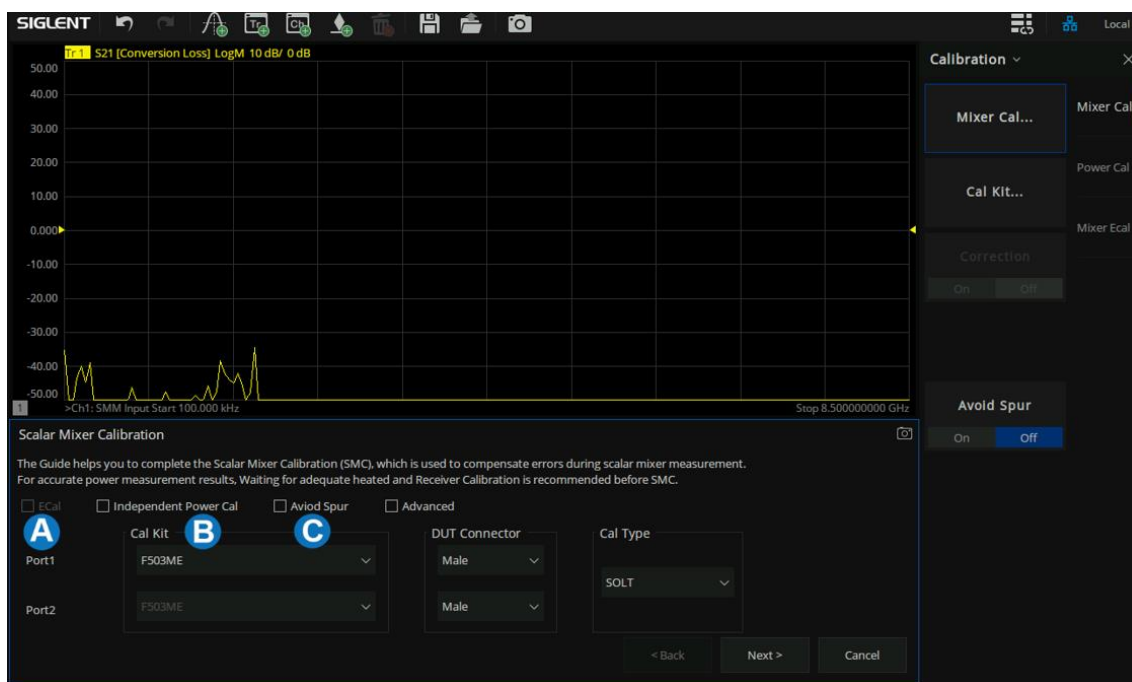
标量混频校准开启界面
