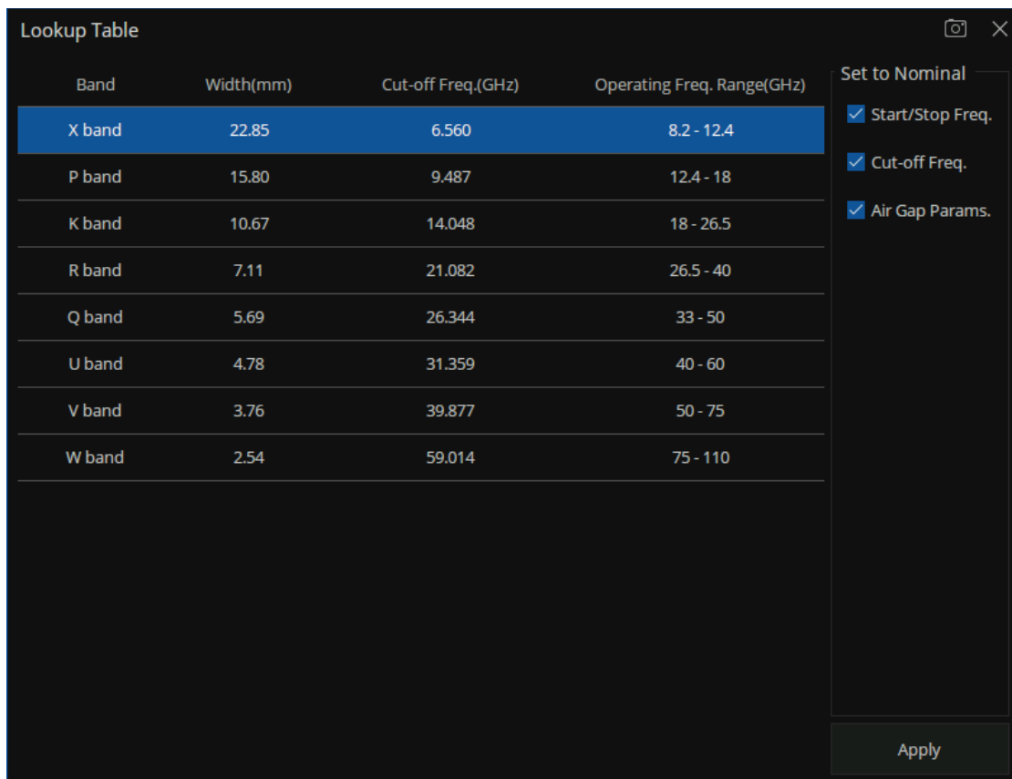
图 15-5 Lookup Table 选项卡
