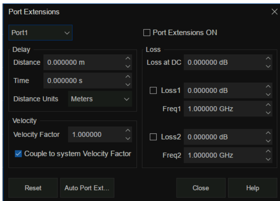
图 7-5 端口延伸设置界面
