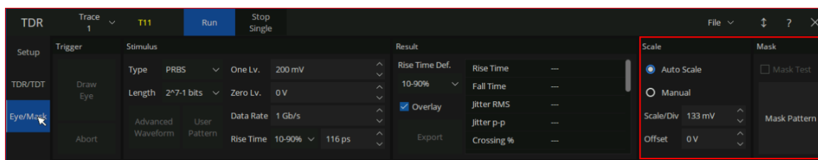
图 10-14 眼图刻度及模板设置
