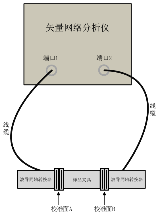
图 15-14 设备连接示意图
