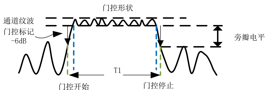
图 8-15 门控示意图
