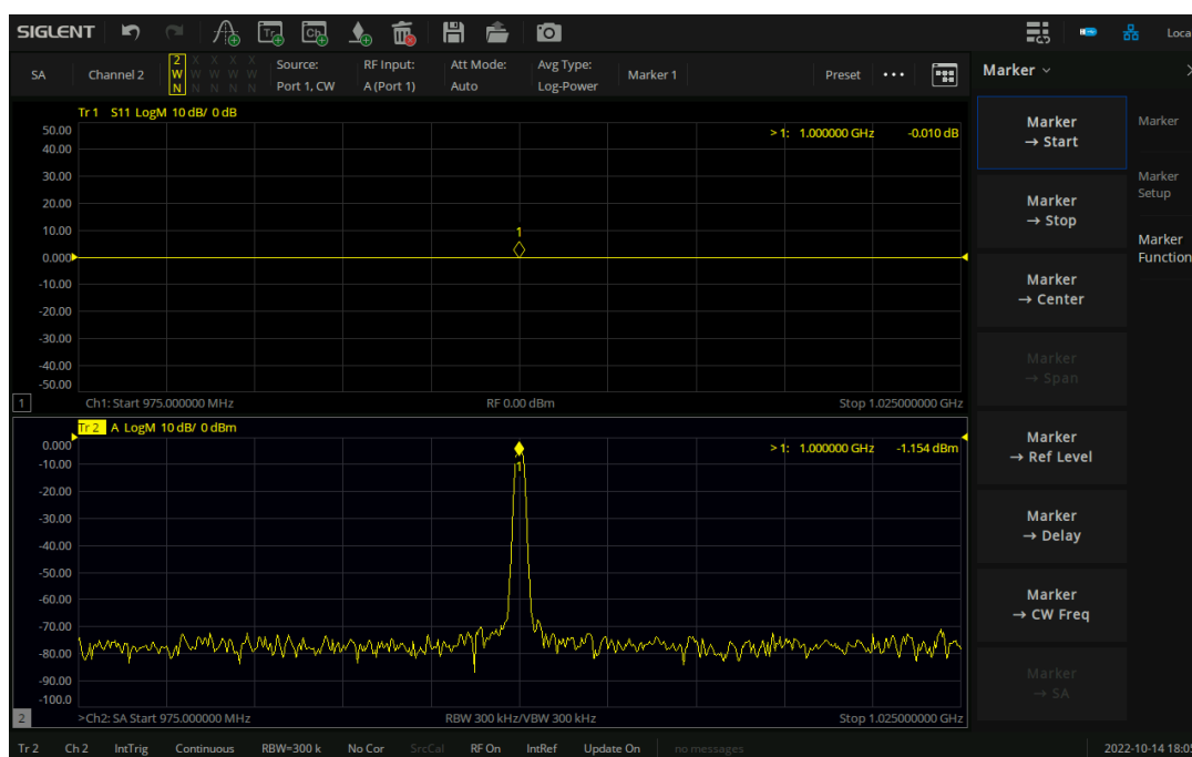
图 11-11-12 Marker → SA 界面
