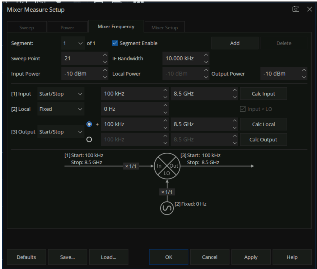
段扫描 SMM Mixer Frequency 选项卡
