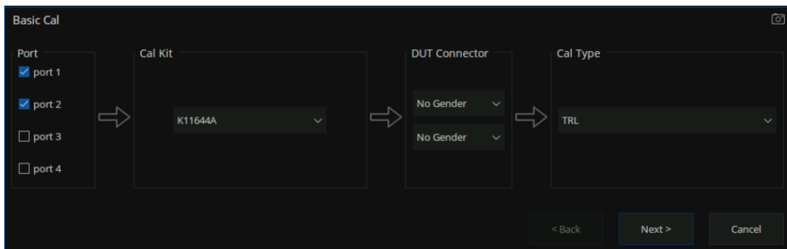
图 15-9 校准向导界面
