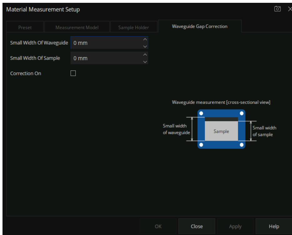
图 15-8 Waveguide Gap Correction 选项卡
