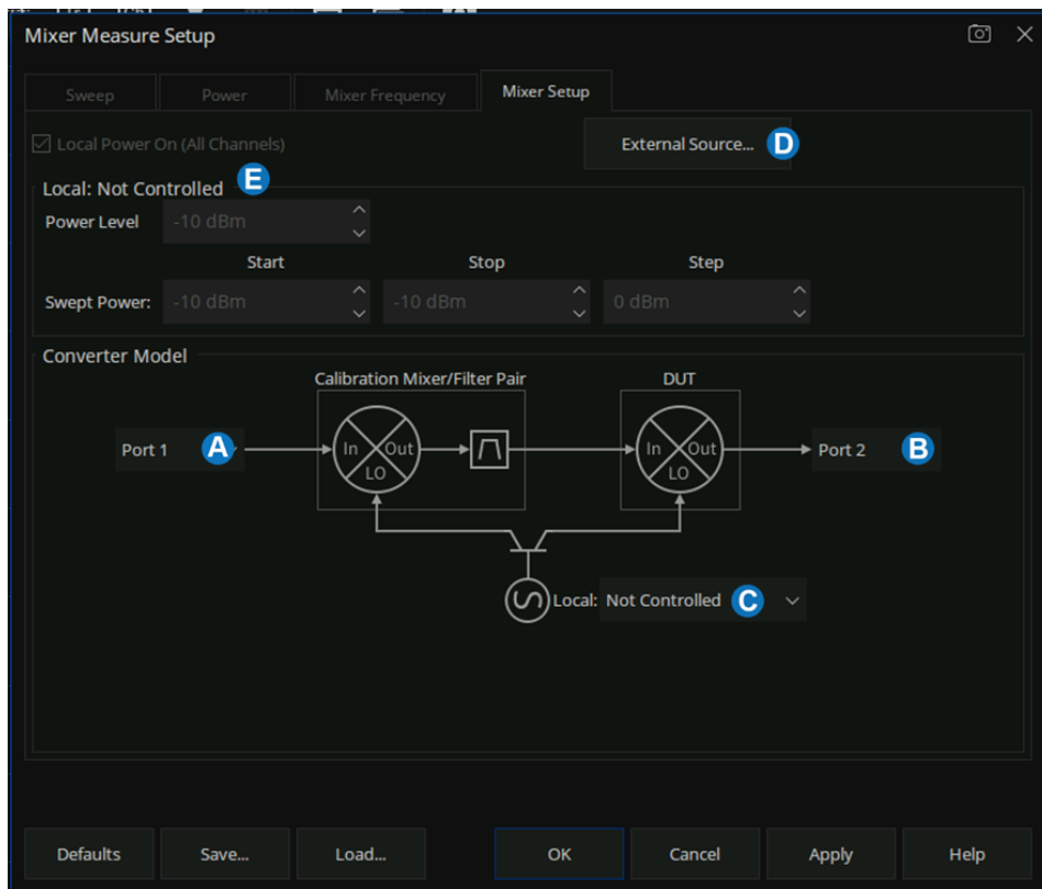
VMM Mixer Setup 选项卡
