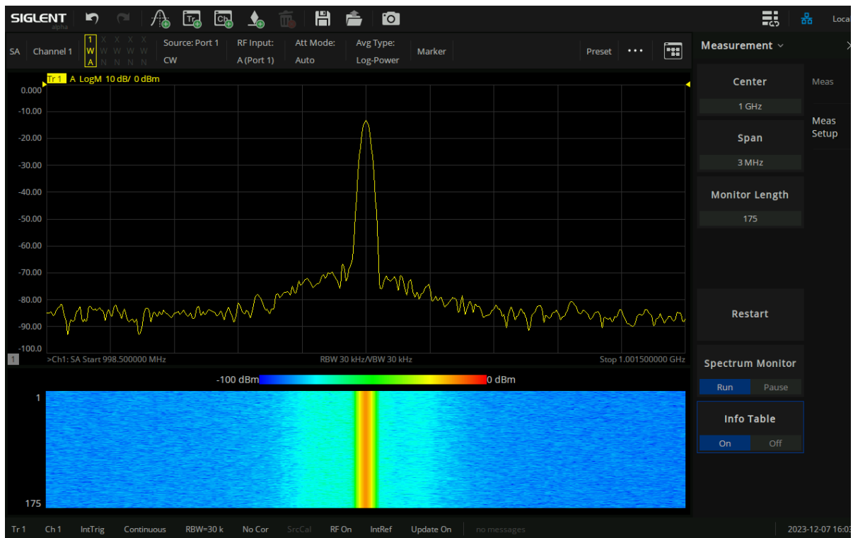
图 11-18 频谱监测测量界面
