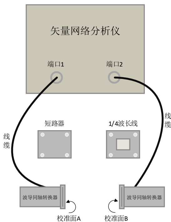
图 15-11 波导校准连接示意图
