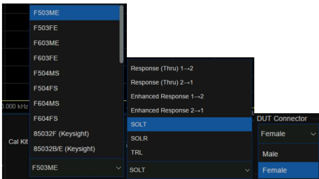
图 7-3 校准向导界面
