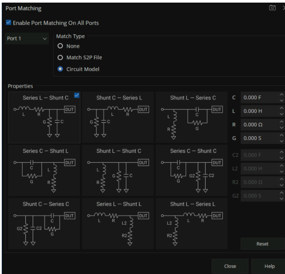
图 7-8 端口匹配
