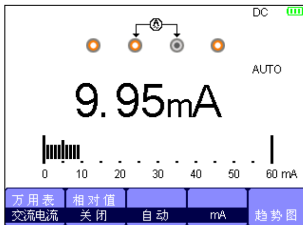
万用表交流电流测量
