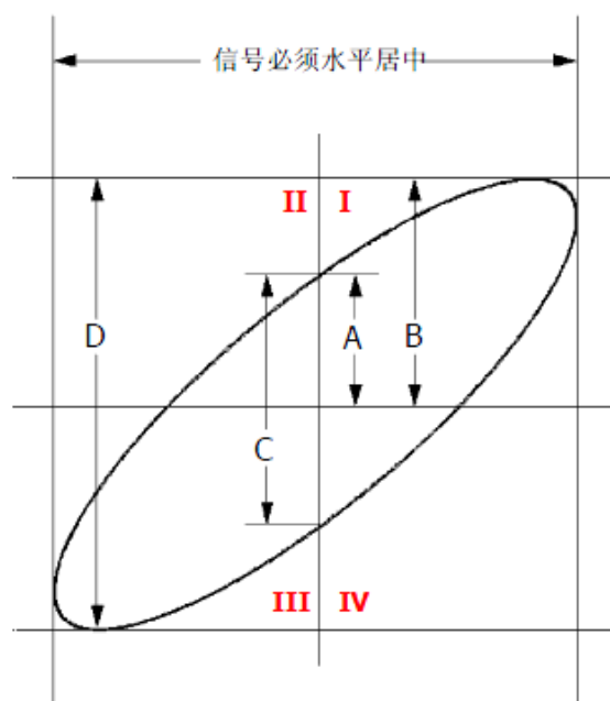
图 26 李沙育测量原理图
