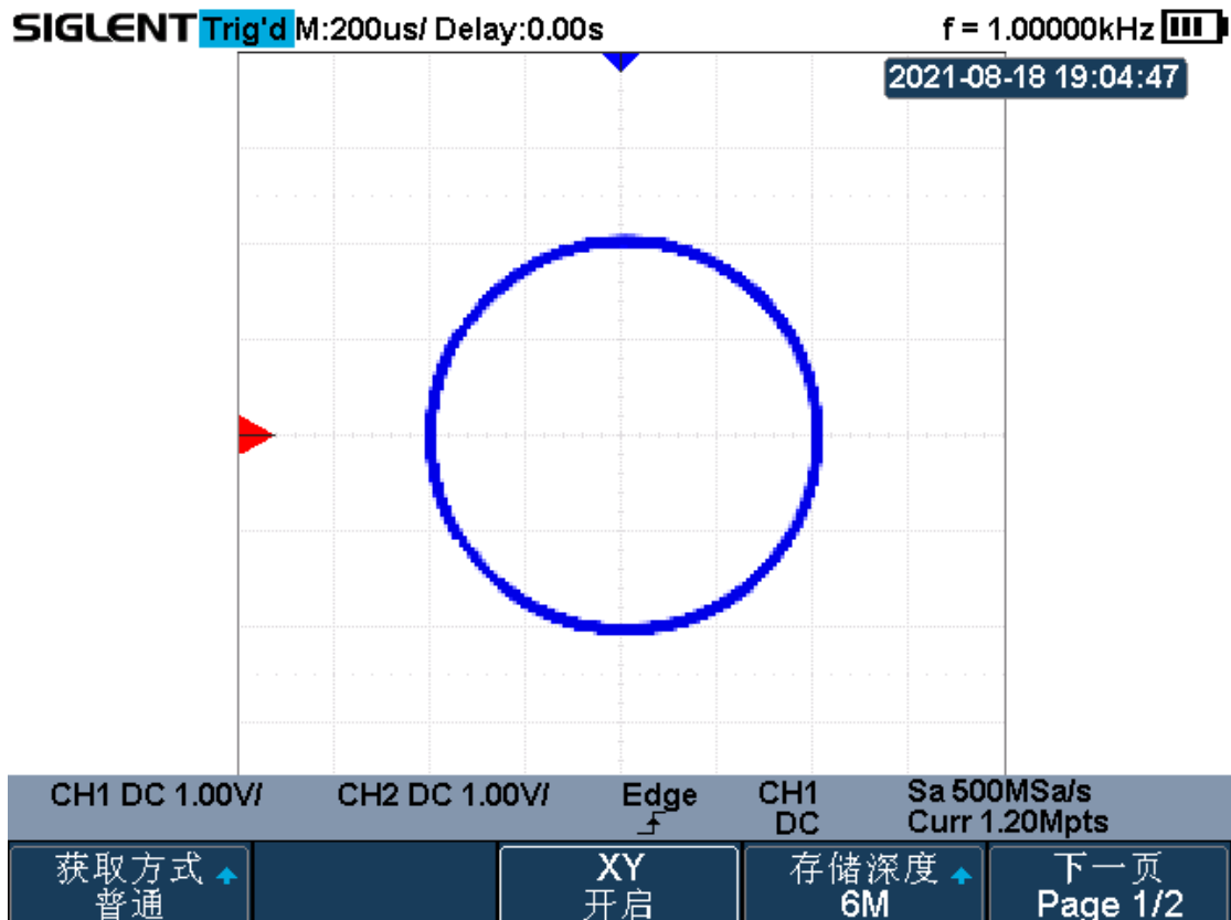
图 27 李沙育测量实例
