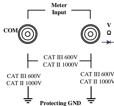
SHS1000X 万用表输入端测量类别示意
