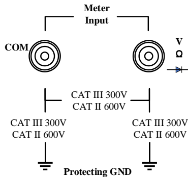
SHS800X 万用表输入端测量类别示意
