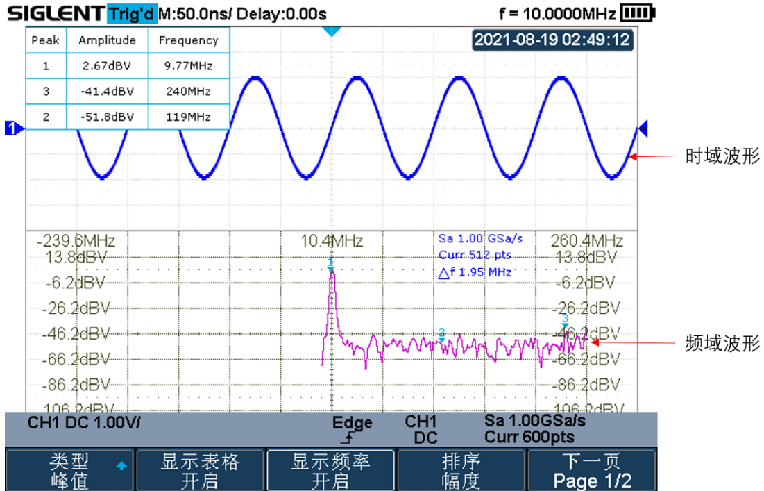
图 86 FFT 波形
