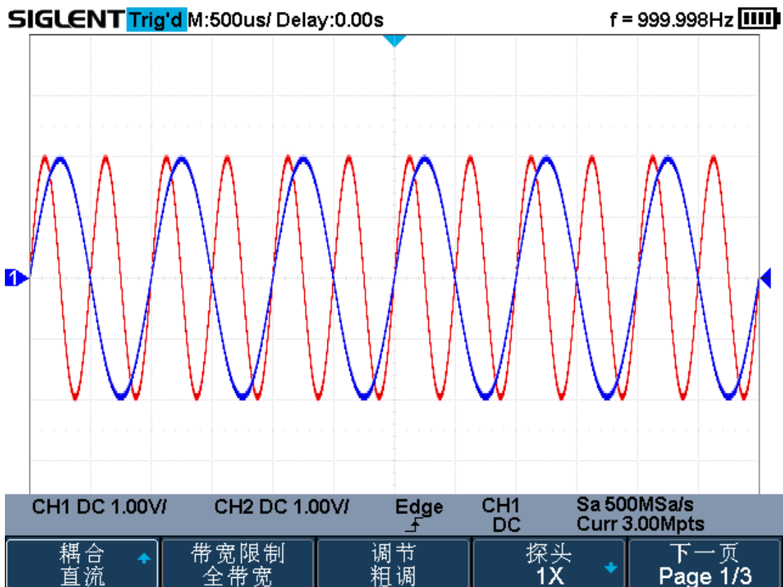
图 14 通道波形图
