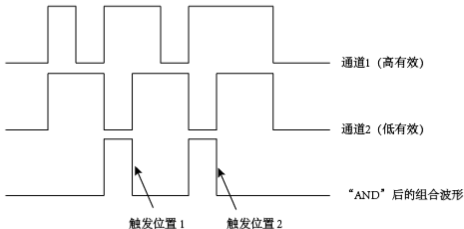
图 42 码型触发示意图
