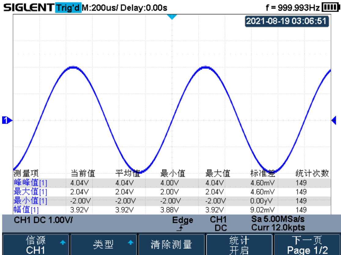
图 97 测量统计
