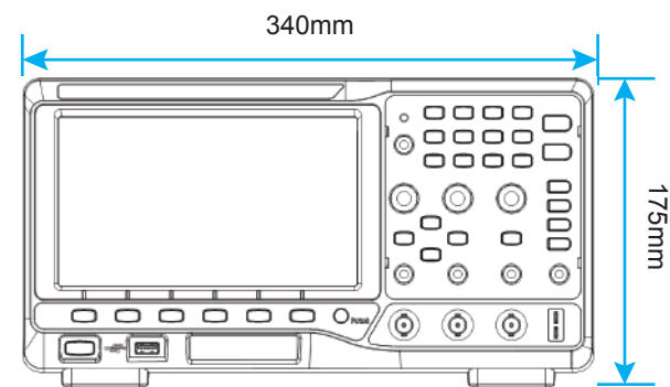
图1 正视图
