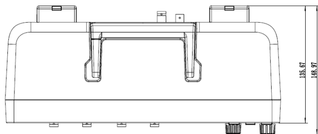
正视图
