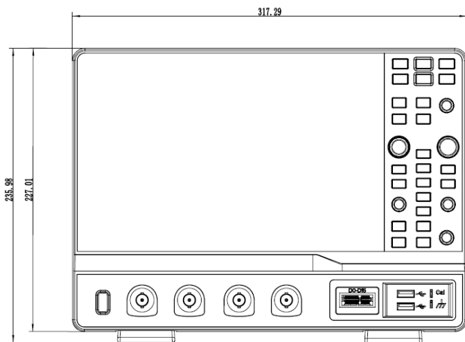
正视图
