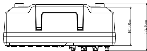
图 2 俯视图
