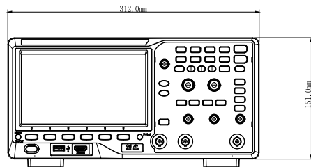
图 1 正视图
