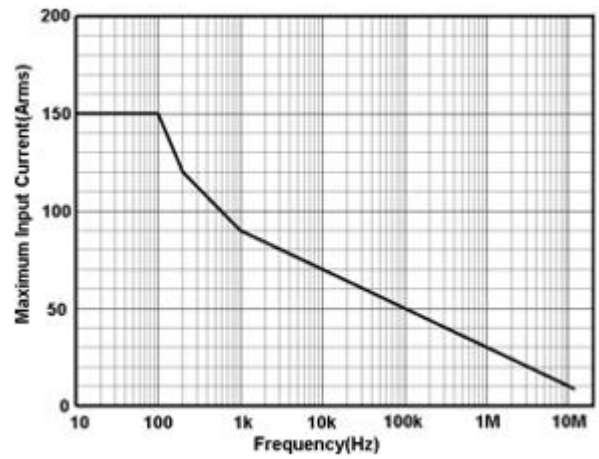
图 5 CP6150 最大测量电流 VS 频率曲线
