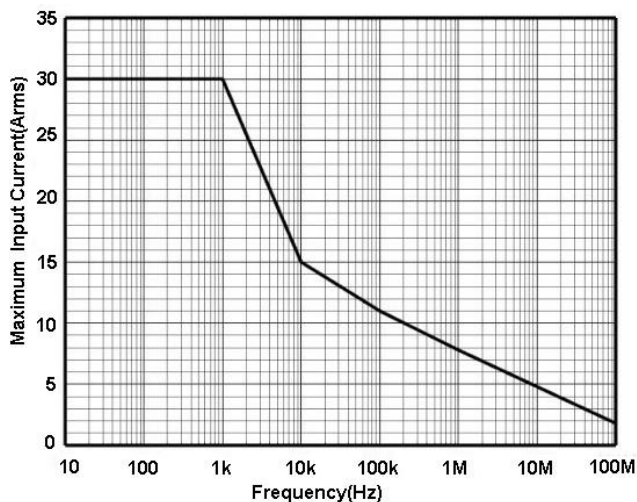
图 2.b CP6030A 最大测量电流 VS 频率曲线
