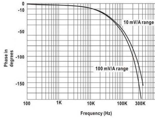
CP4070A 1A 峰值时典型的相位与频率对应图
