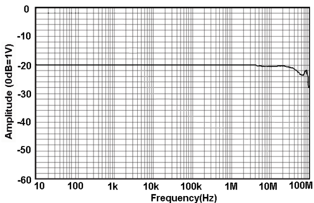
图 1 .a CP6030 幅频曲线
