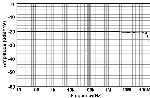
图 1 .b CP6030A 幅频曲线
