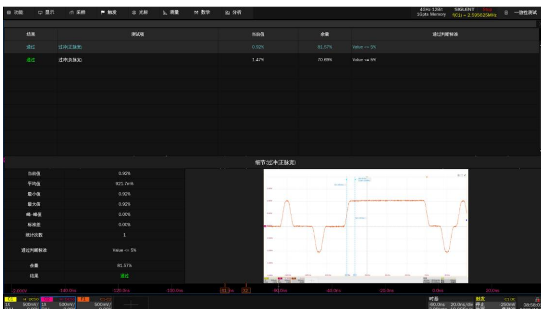
图 6-8 过冲测试项目
