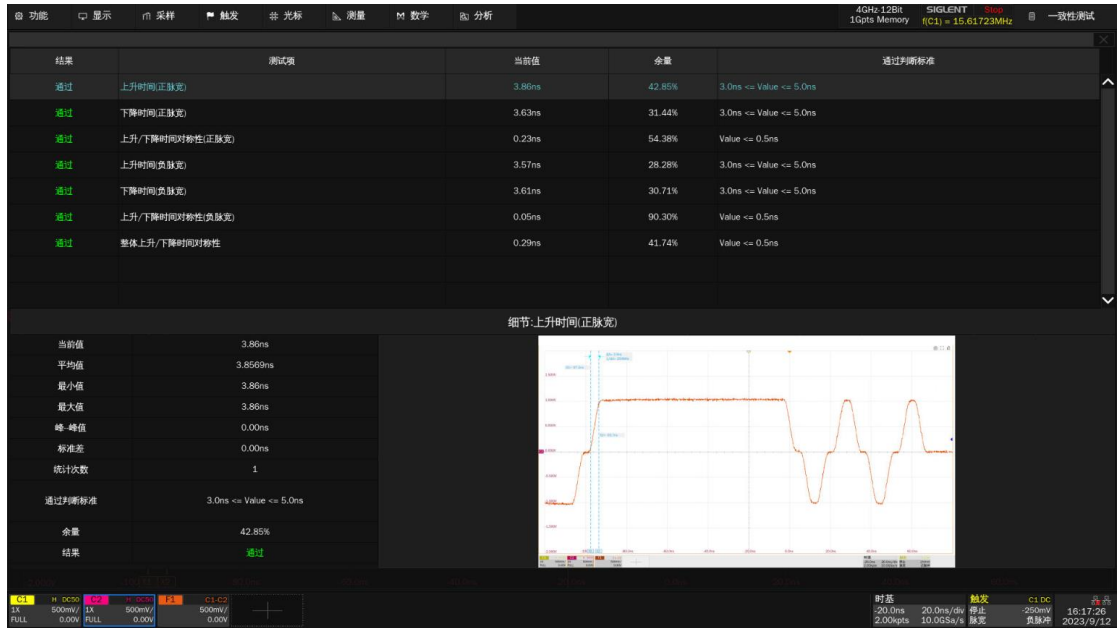
图 6-10 上升/下降时间测试列表
